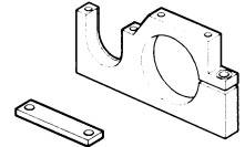
ST-P08 Antivibration Motor Mount (Machine Cut) 진동방지 모터 마운트
