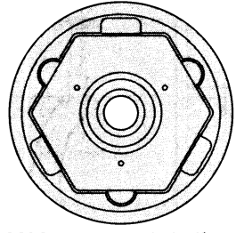
MA25 ×2 デフハウジング Diff housing Differential-Gehäuse Logement de différentiel
