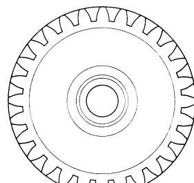
MC5 x2 リングギヤ Ring gear Tellerrad Couronne 9445933
